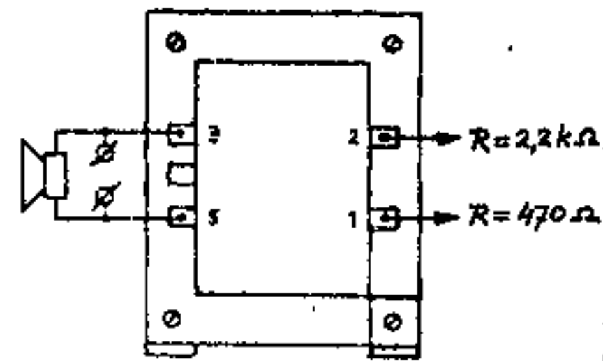
GELUID UITGANGS TRAFU SOUND OUTPUT TRANSF. TONAUSG. ÜBERTRAGER 50 051 581
