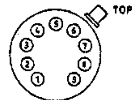
OVERIGE BUIZEN OTHER TUBES ÜBRIGE RÖHREN
