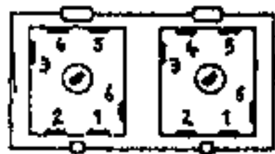
BEELD MF. TRAFU 1, 2, 3, 4 PICTURE IF. TRANSF. BILDZF. ÜBERTRAGER AT 2023 50 051 709
