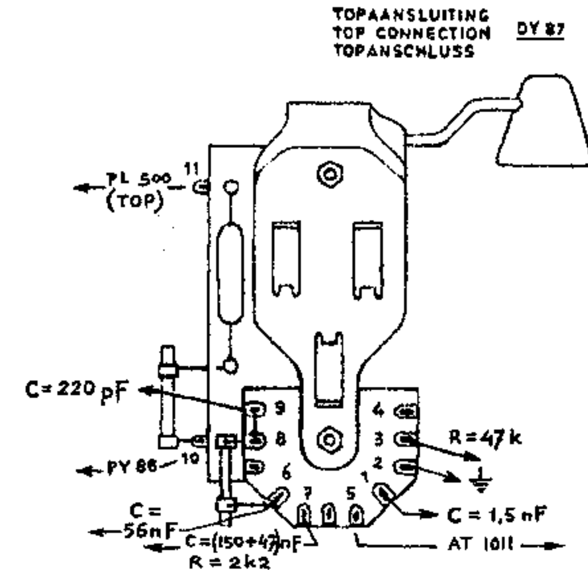
LIJNUITGANGS TRAFU LINE OUTPUT TRANSF. ZEILEN AUSG. ÜBERTRAGER AT 2023 50 051 709
